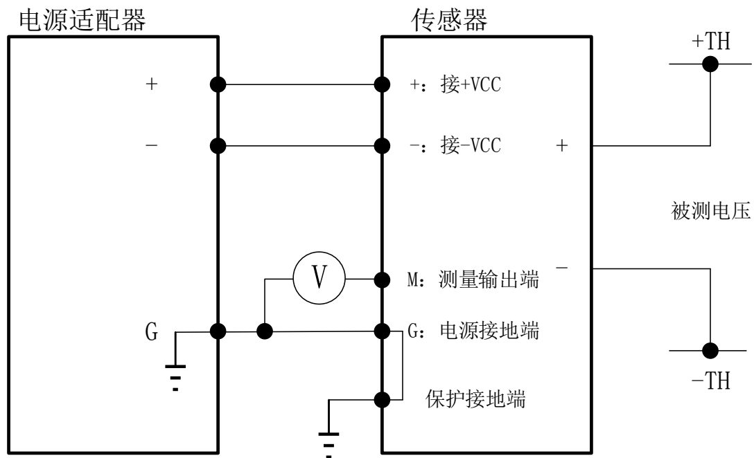
图 3 电气连接图
