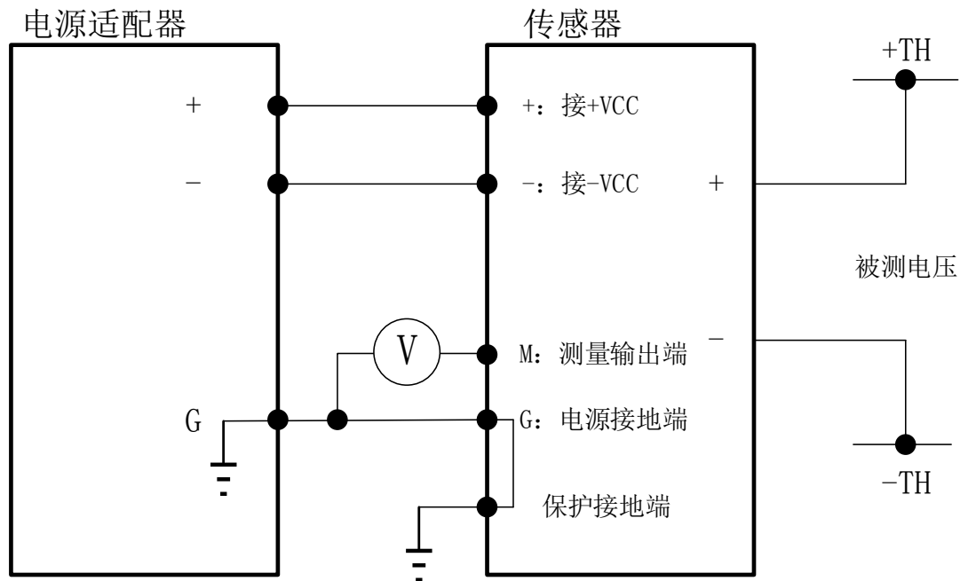
图 3 电气连接图
