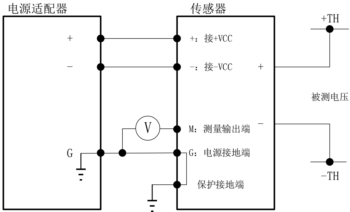
图 3 电气连接图
