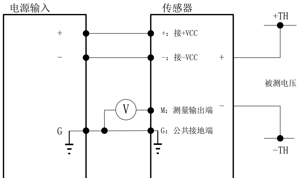
图 2 电气连接图
