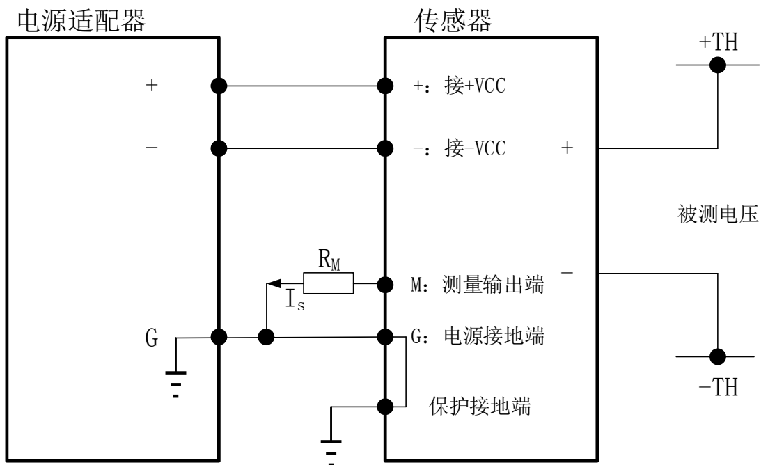
图 3 电气连接图
