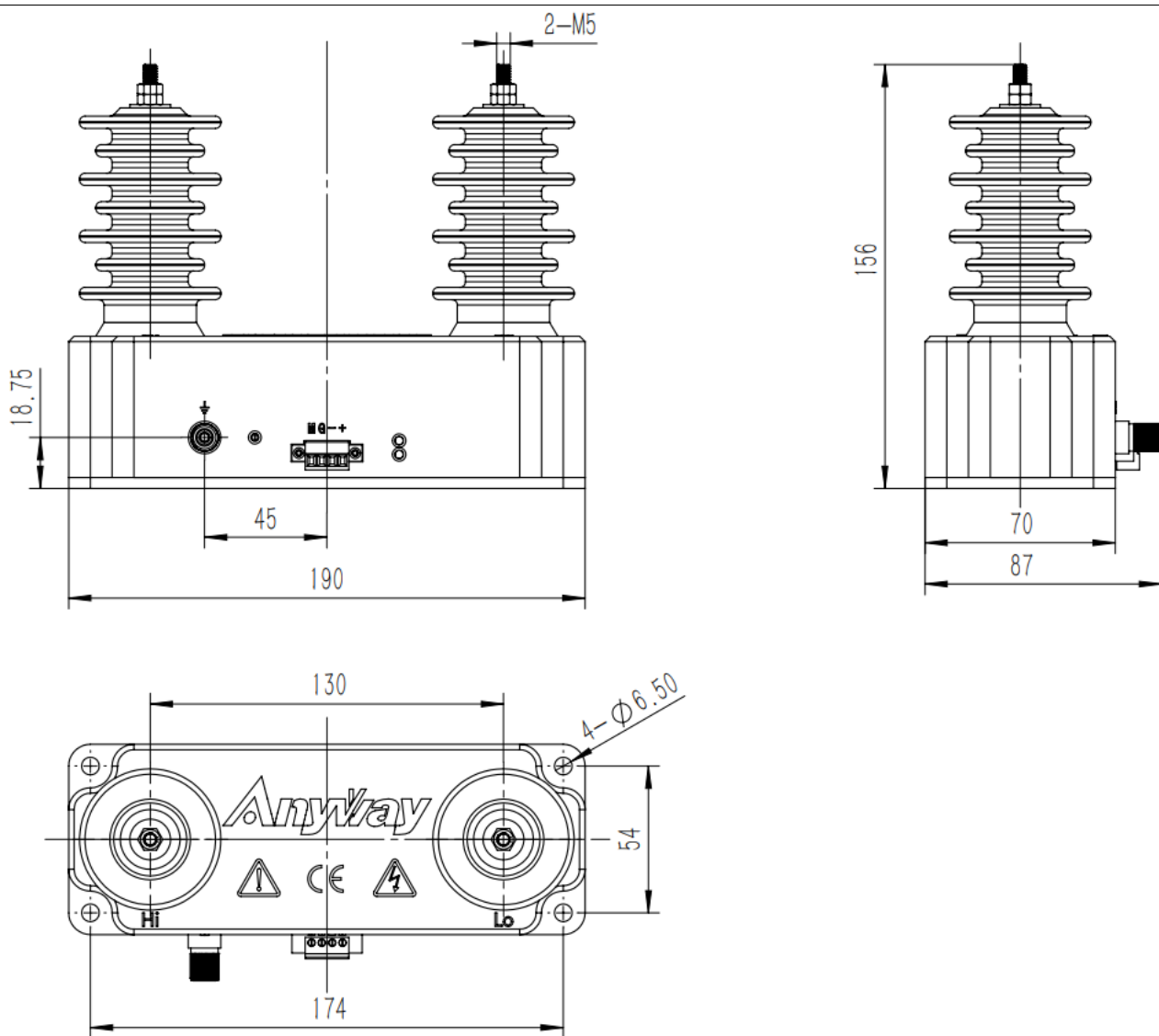
图 1 外形图
