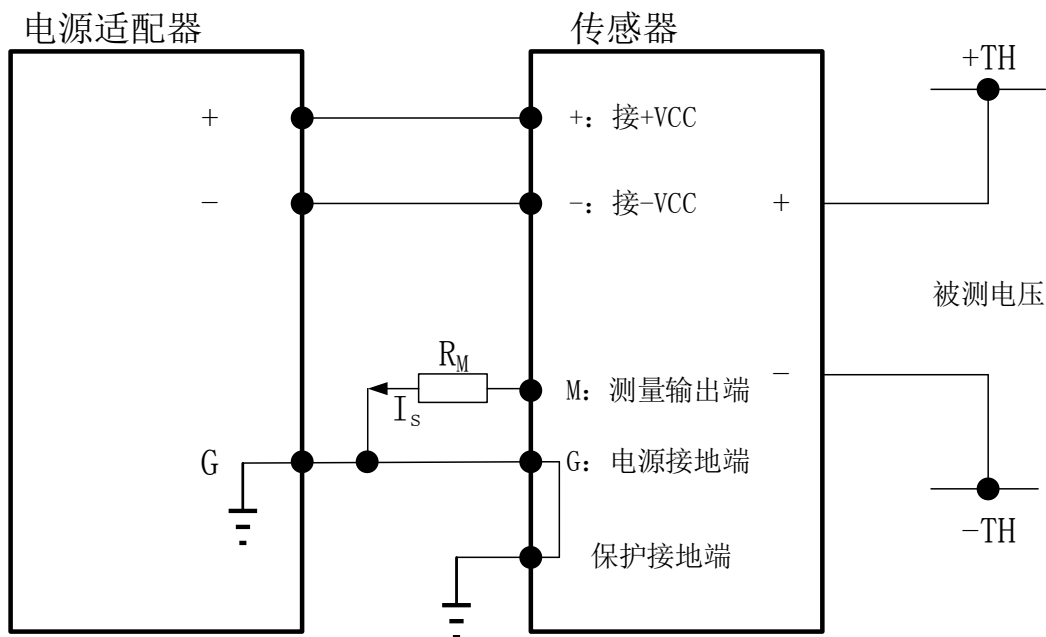
图 3 电气连接图
