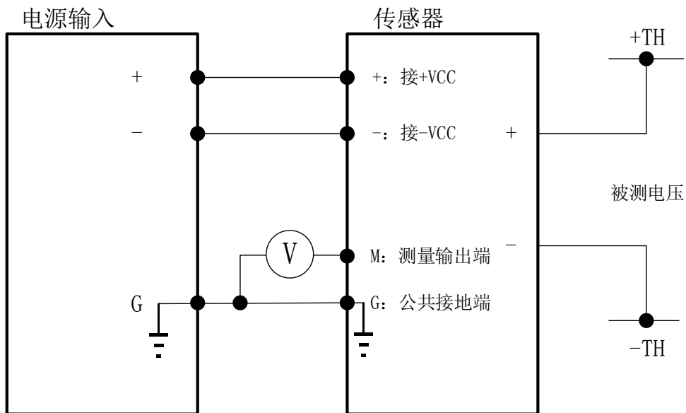
图 2 电气连接图
