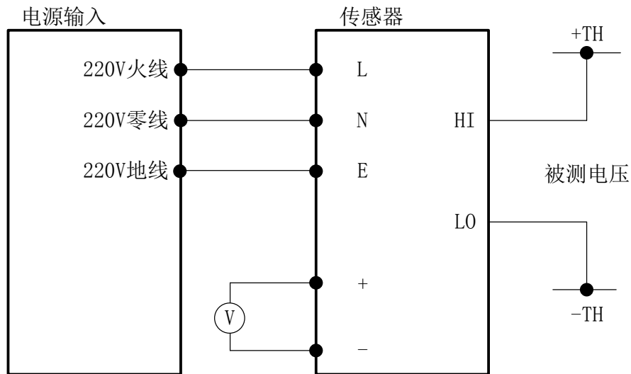
图 2 电气连接图
