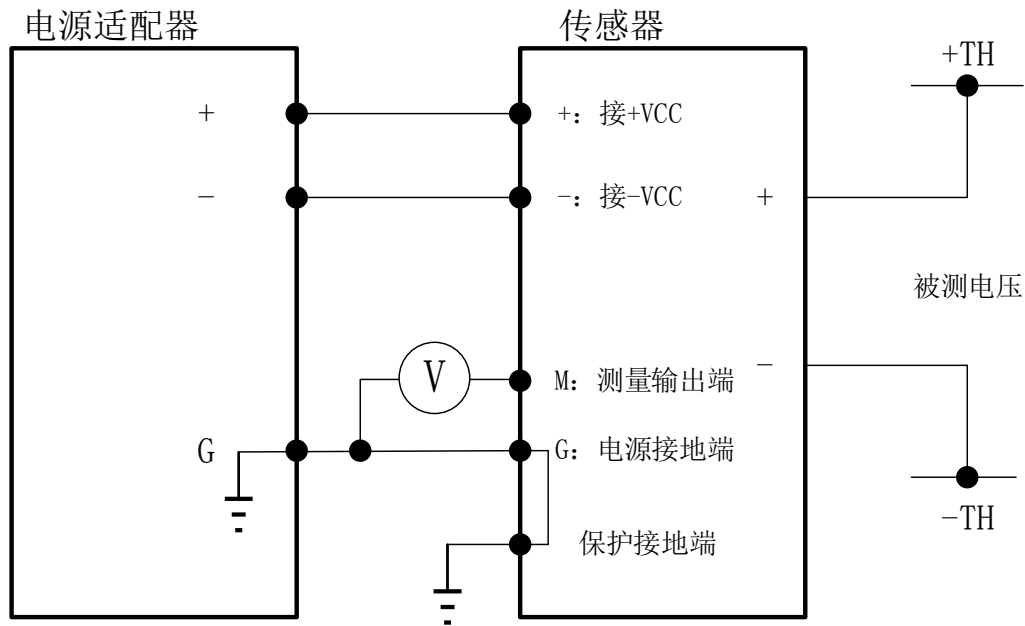
图 3 电气连接图
