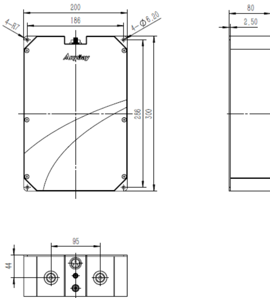
图 1 外形图
