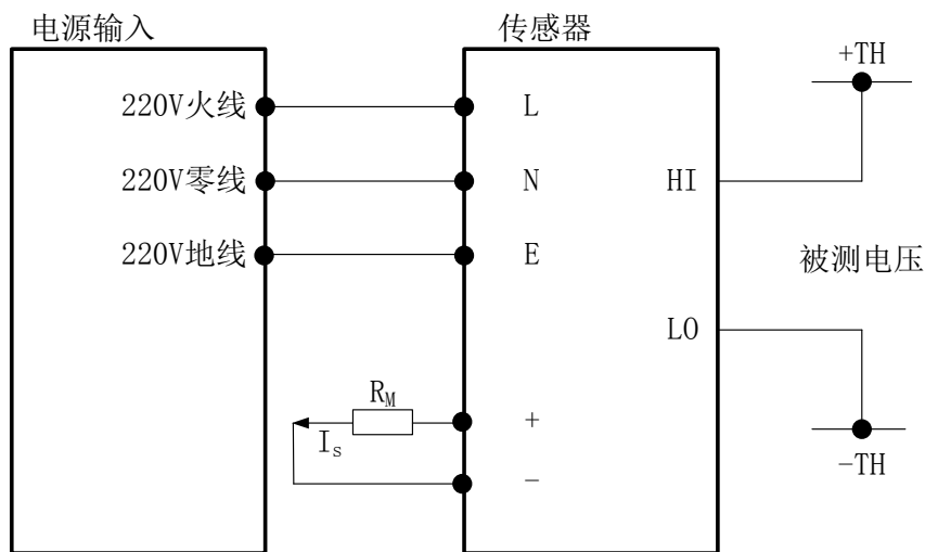
图 3 电气连接图
